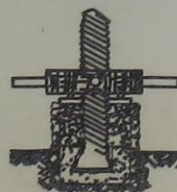
מכש היין של בורג מקובע אחד (ממוקם במרכז משטחי הדריכה של גתות)
