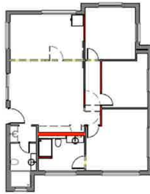
2 קומת קרקע- בניה והריסה 1:100
